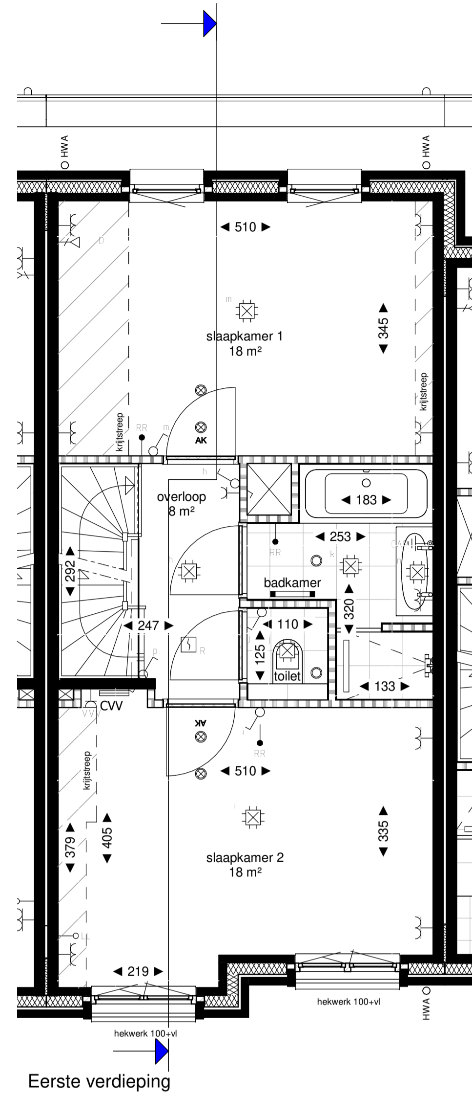
Eerste verdieping
