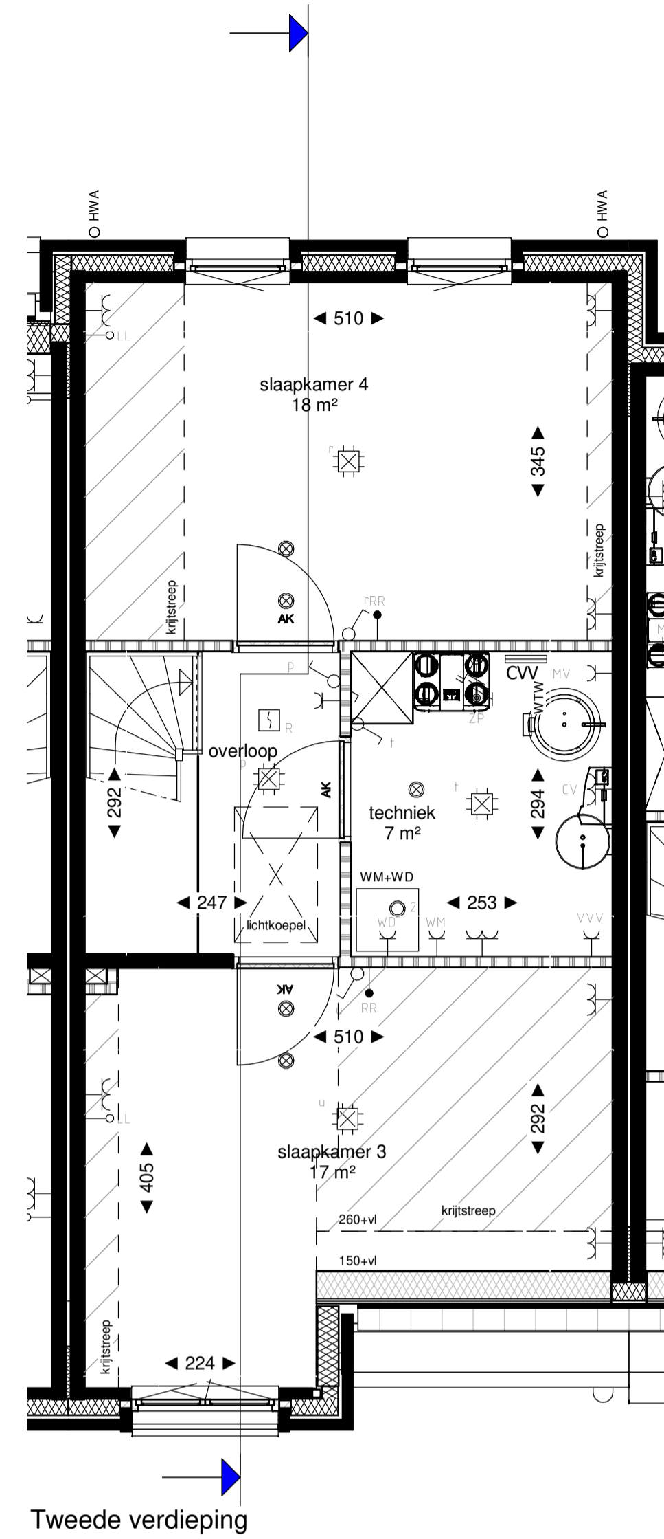
Tweede verdieping
