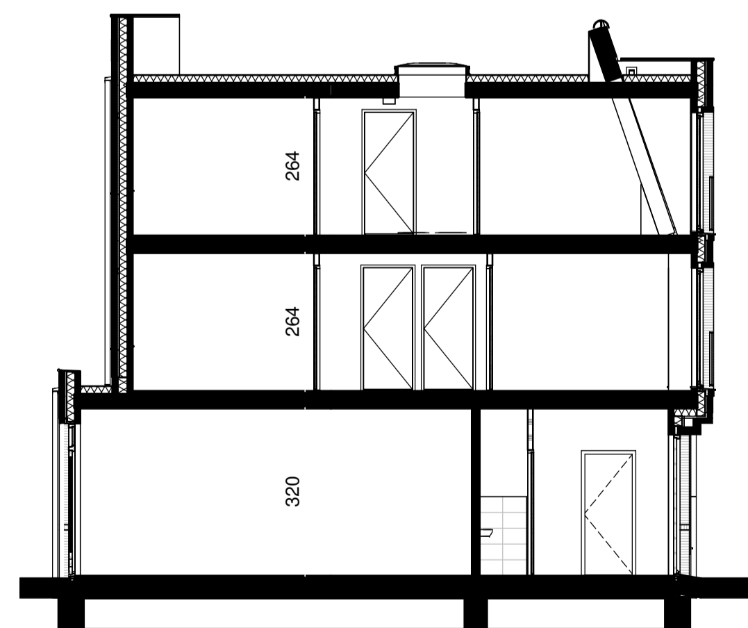
Doorsnede
