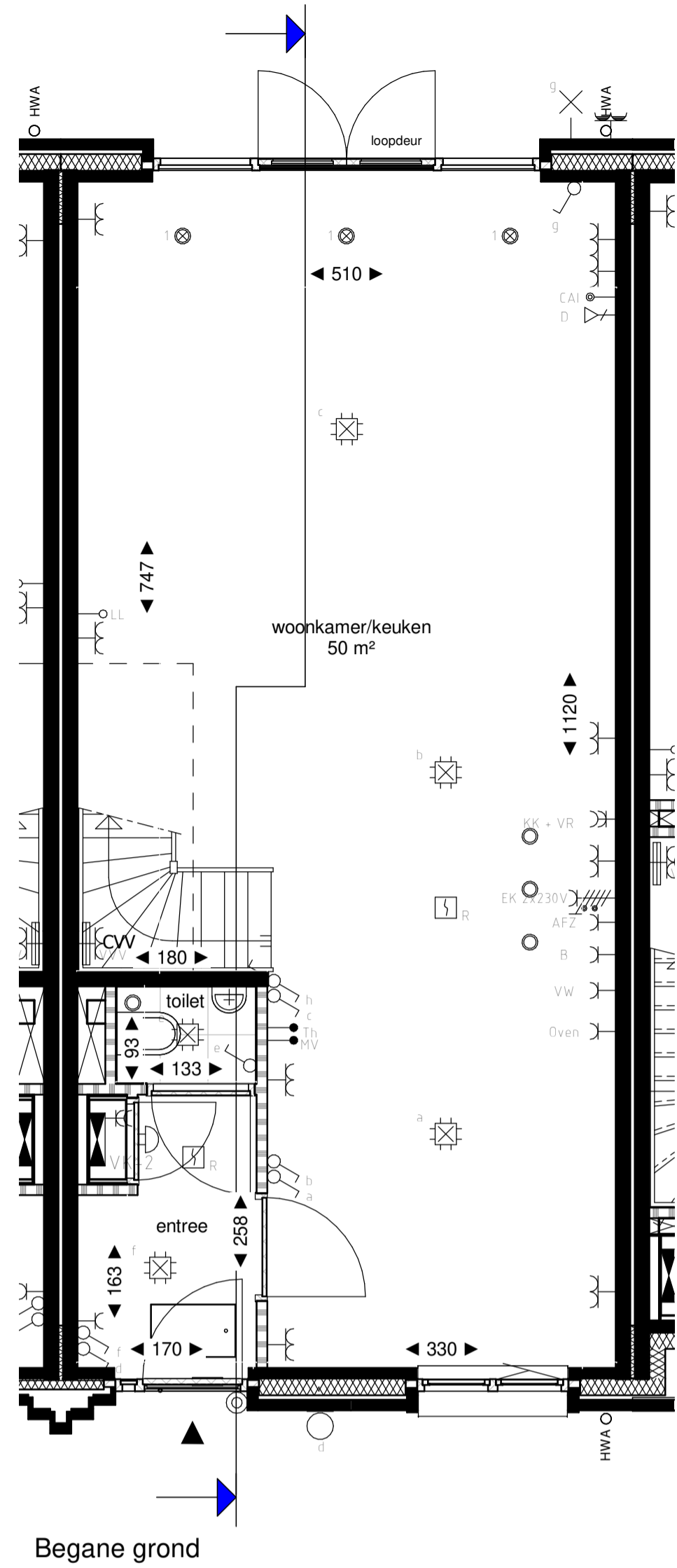
Begane grond
