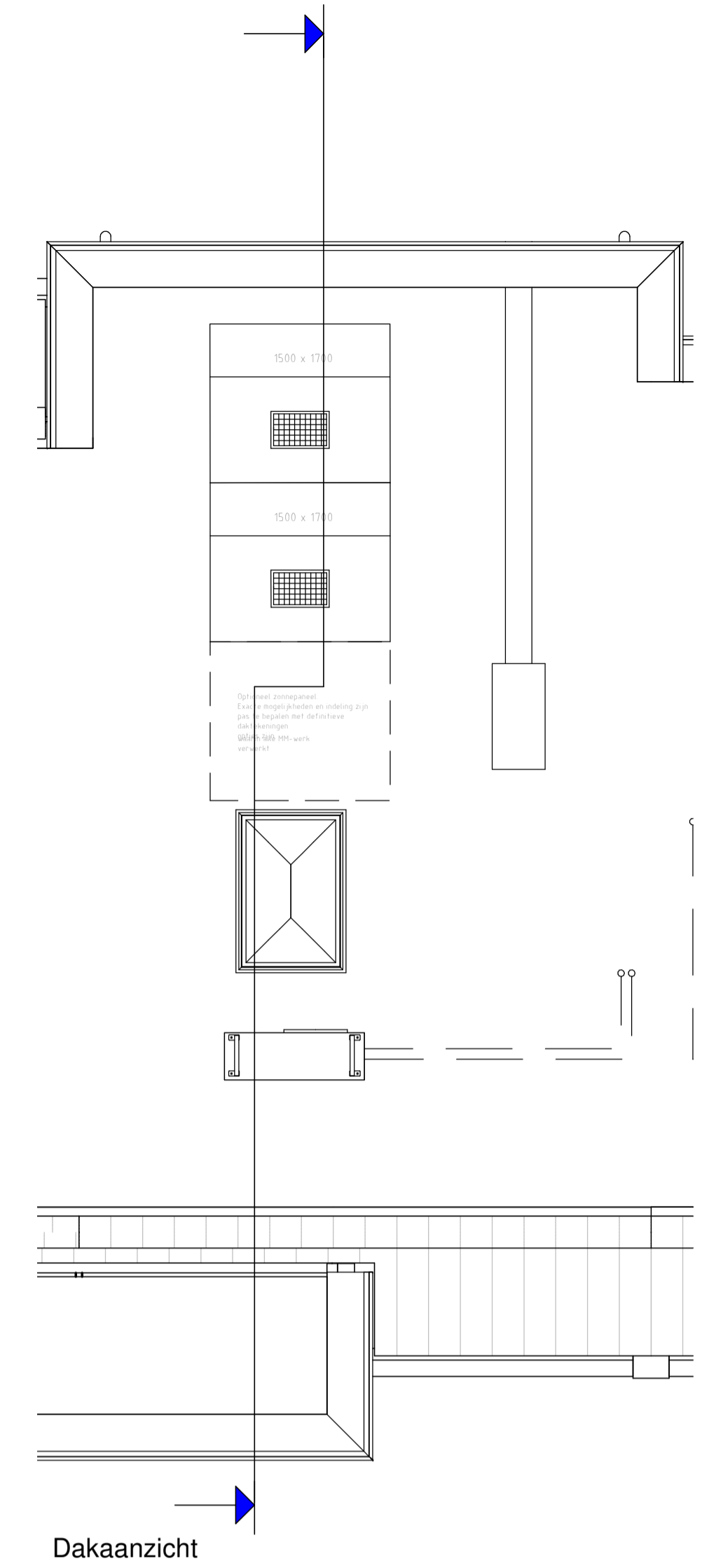
Dakaanzicht
