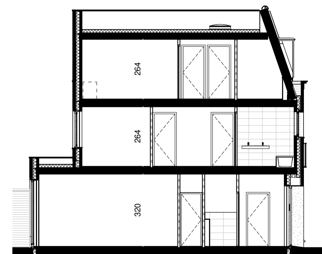
Doorsnede
