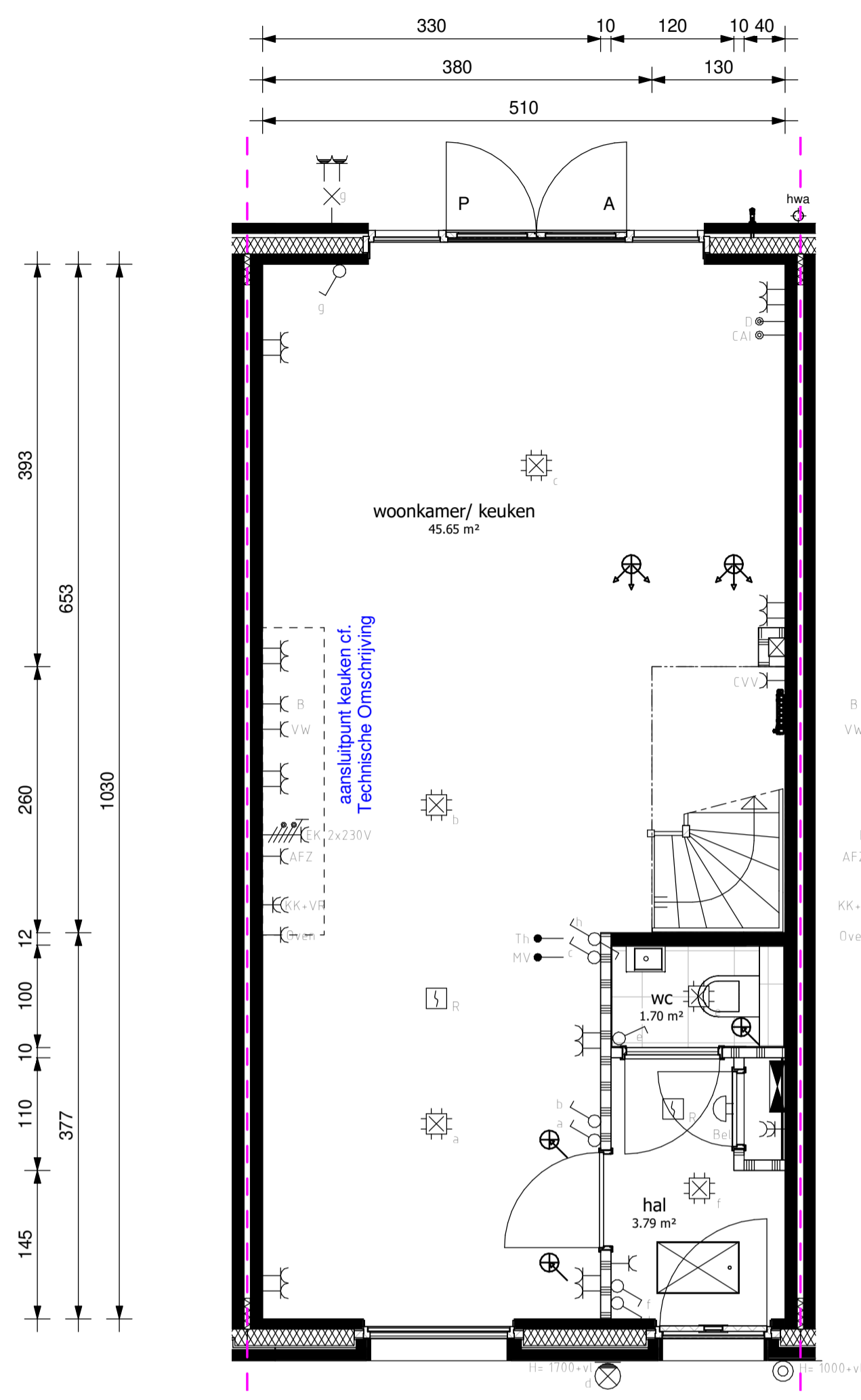
begane grond
