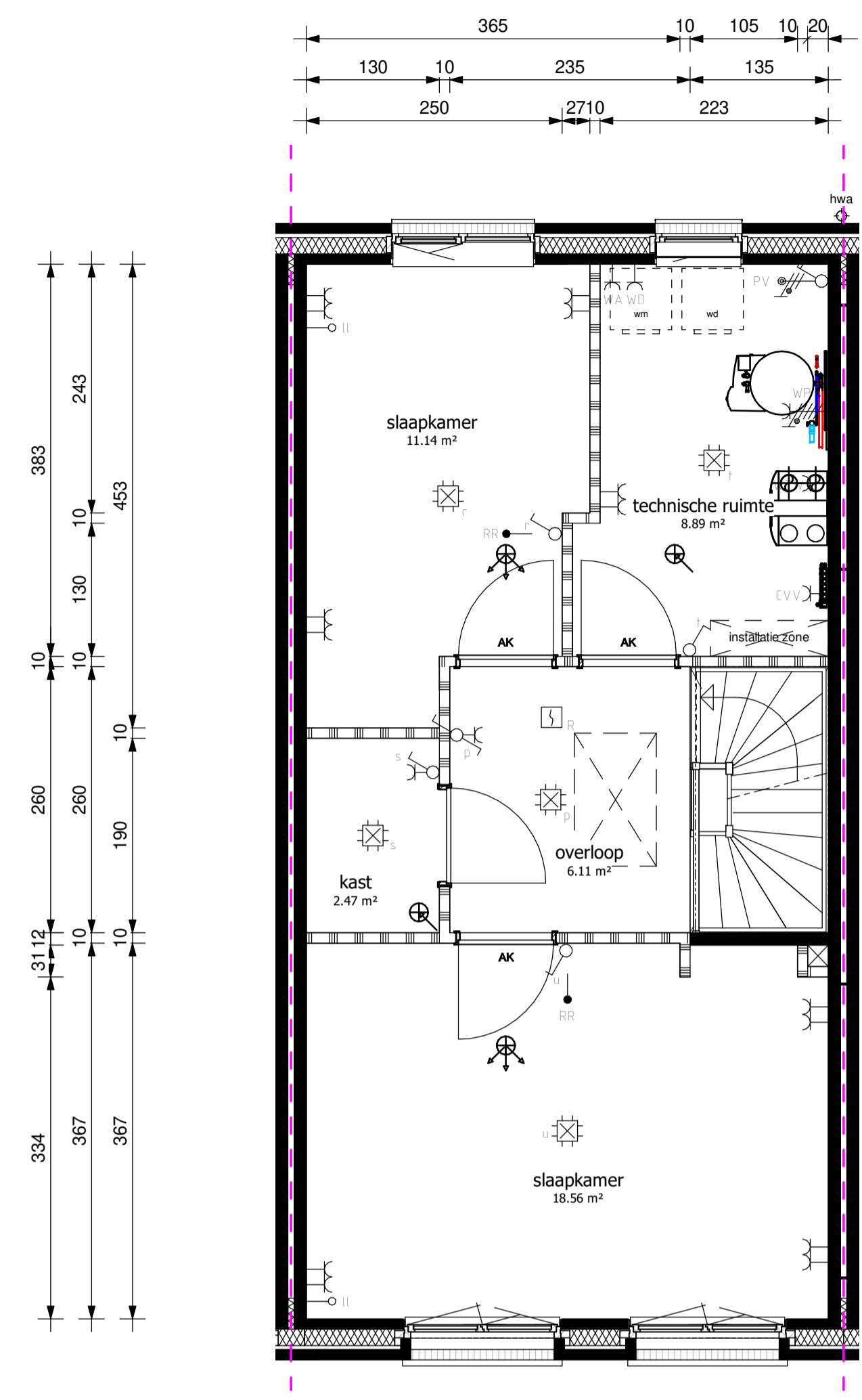
tweede verdieping
