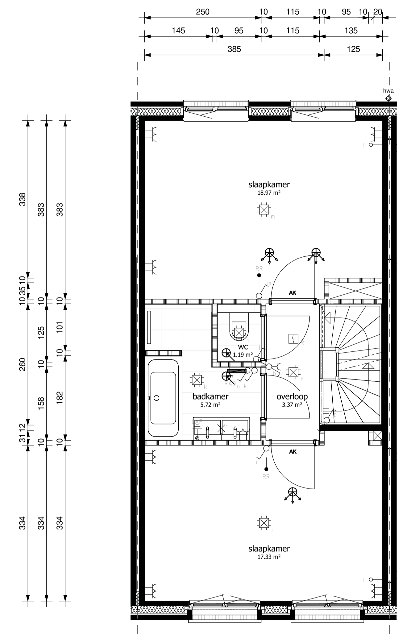
eerste verdieping
