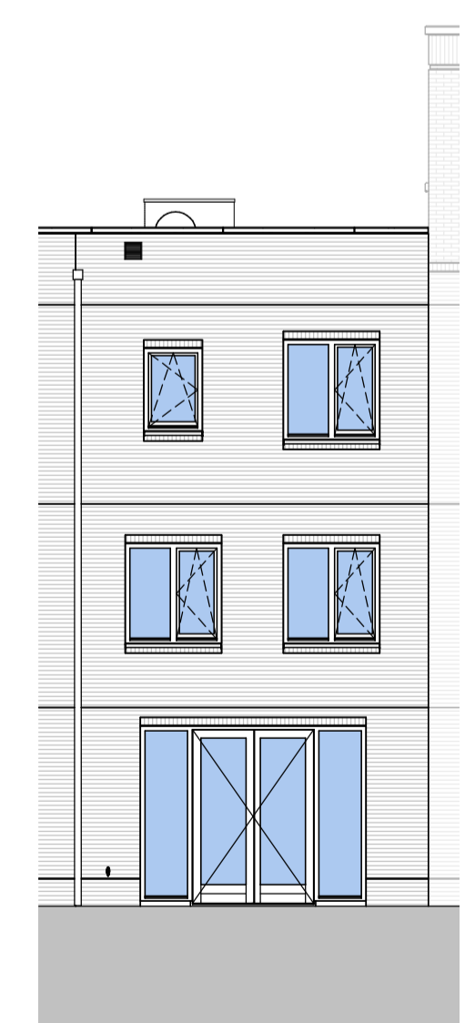
achtergevel
