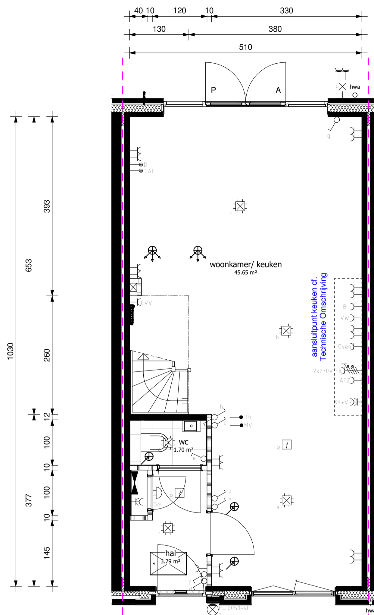
begane grond
