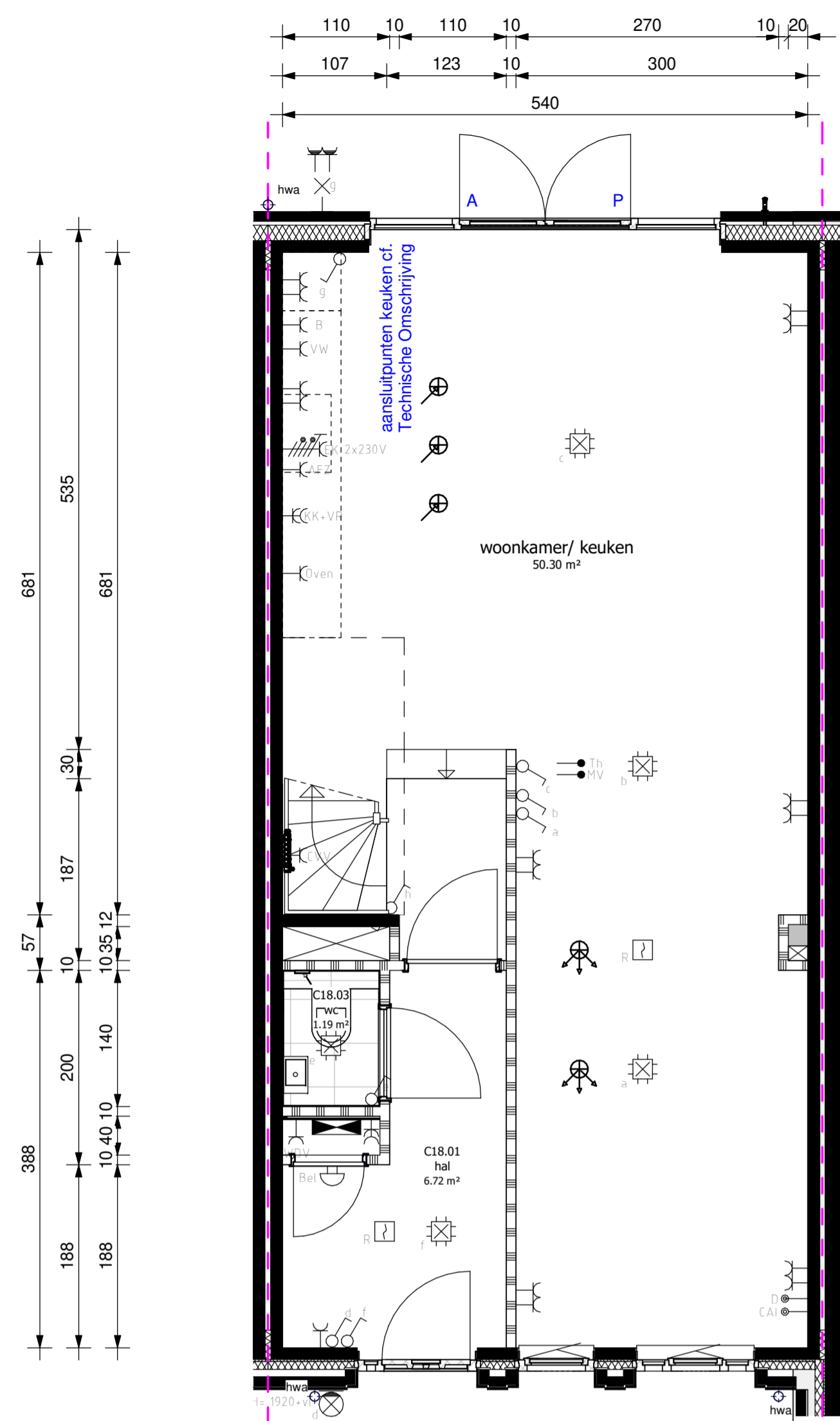
begane grond
