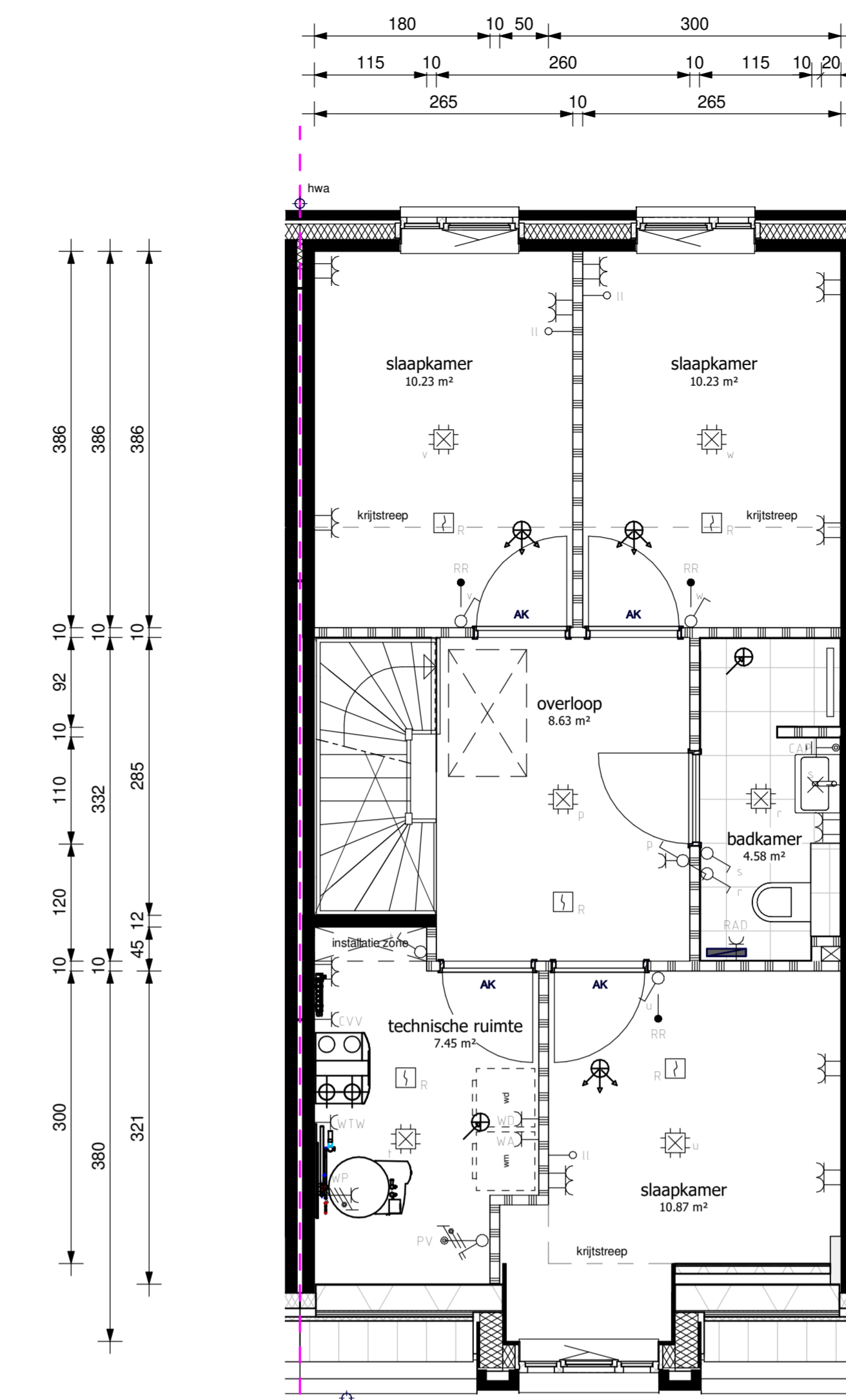
derde verdieping
