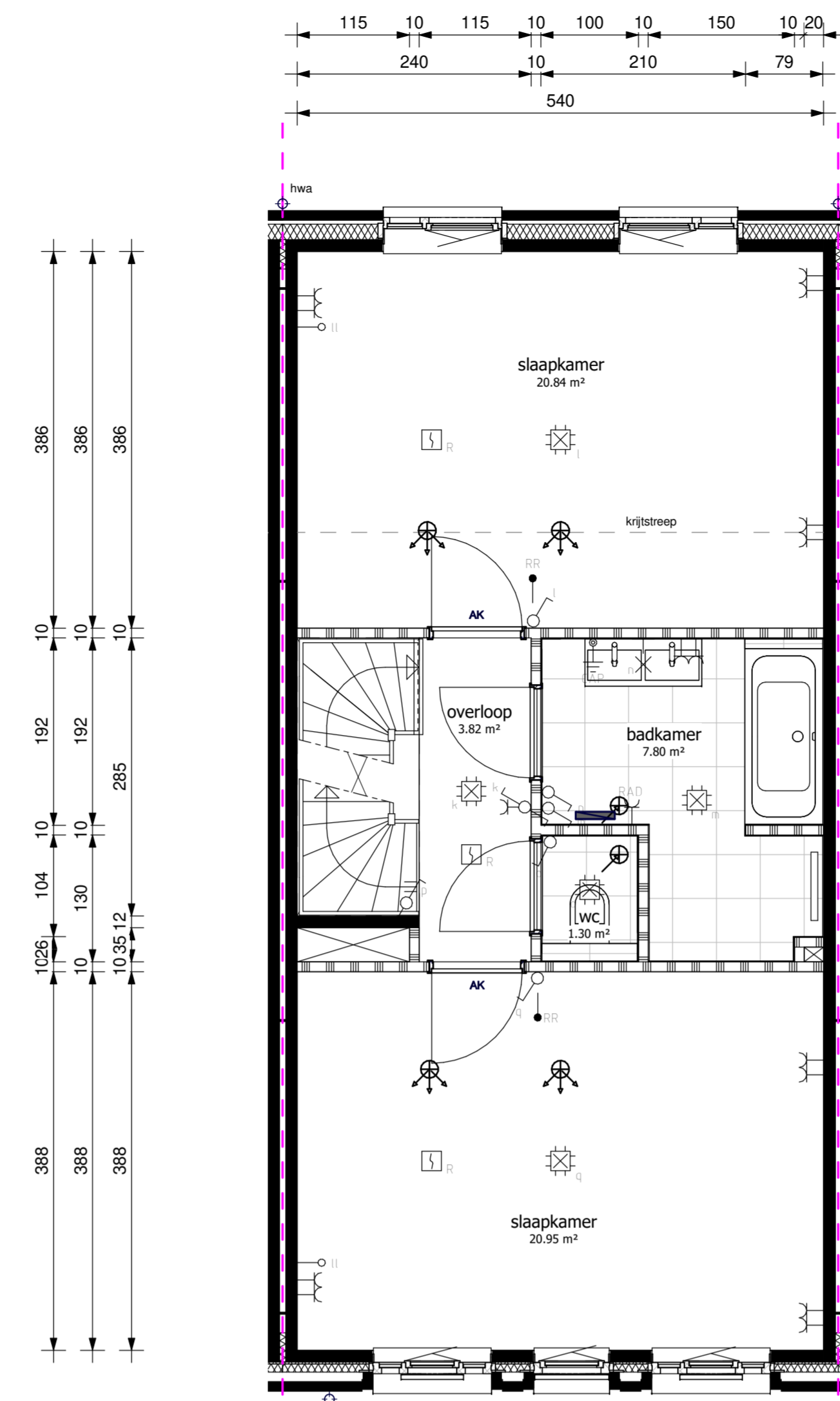
tweede verdieping
