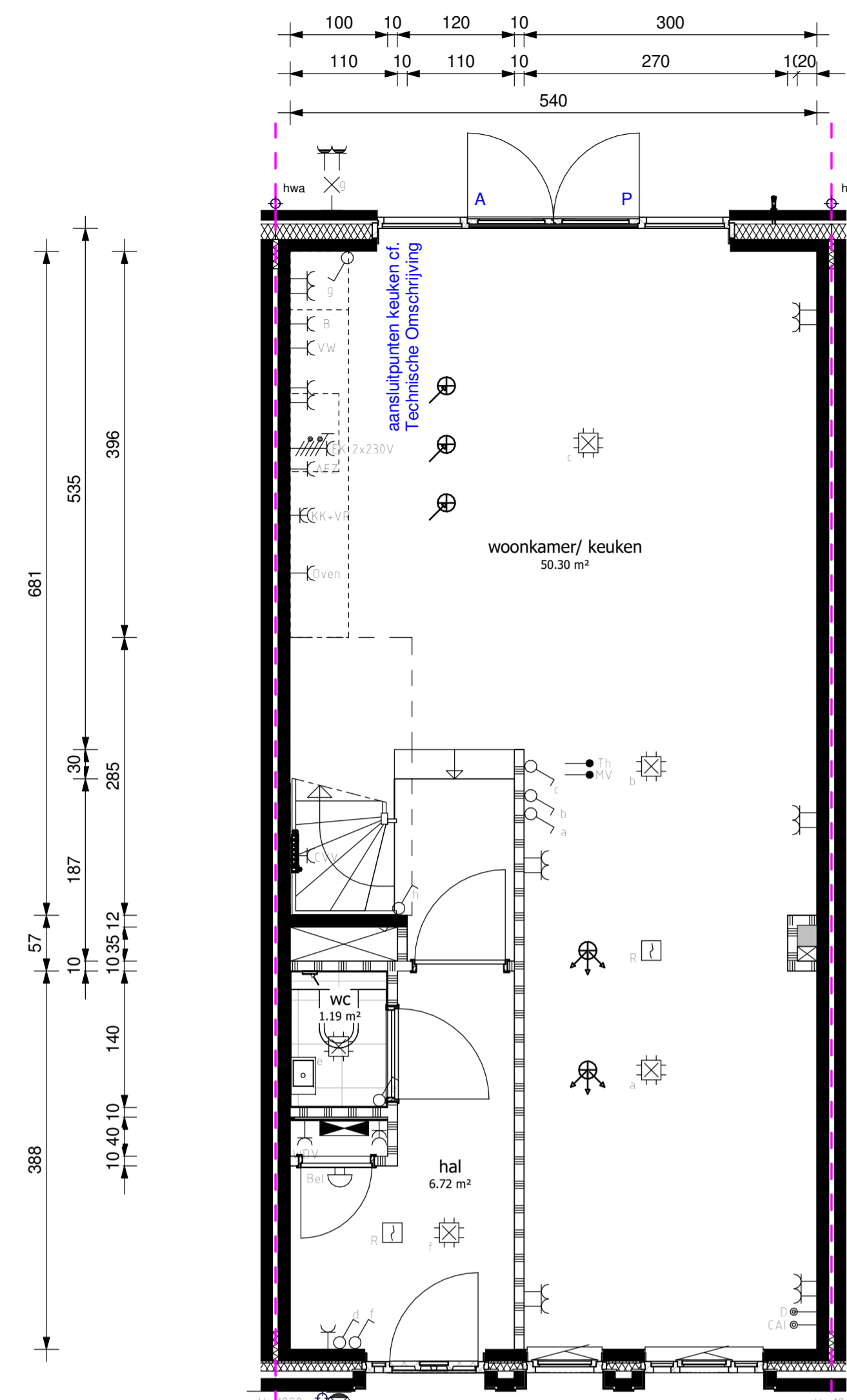
begane grond
