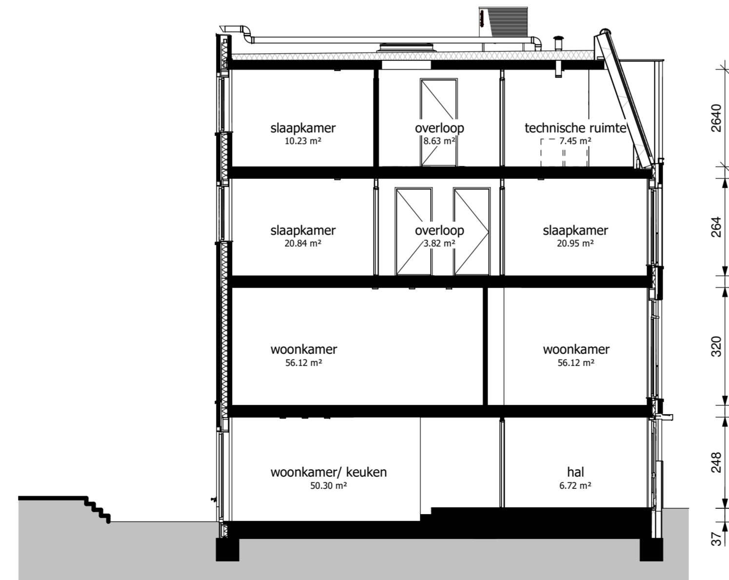
doorsnede
