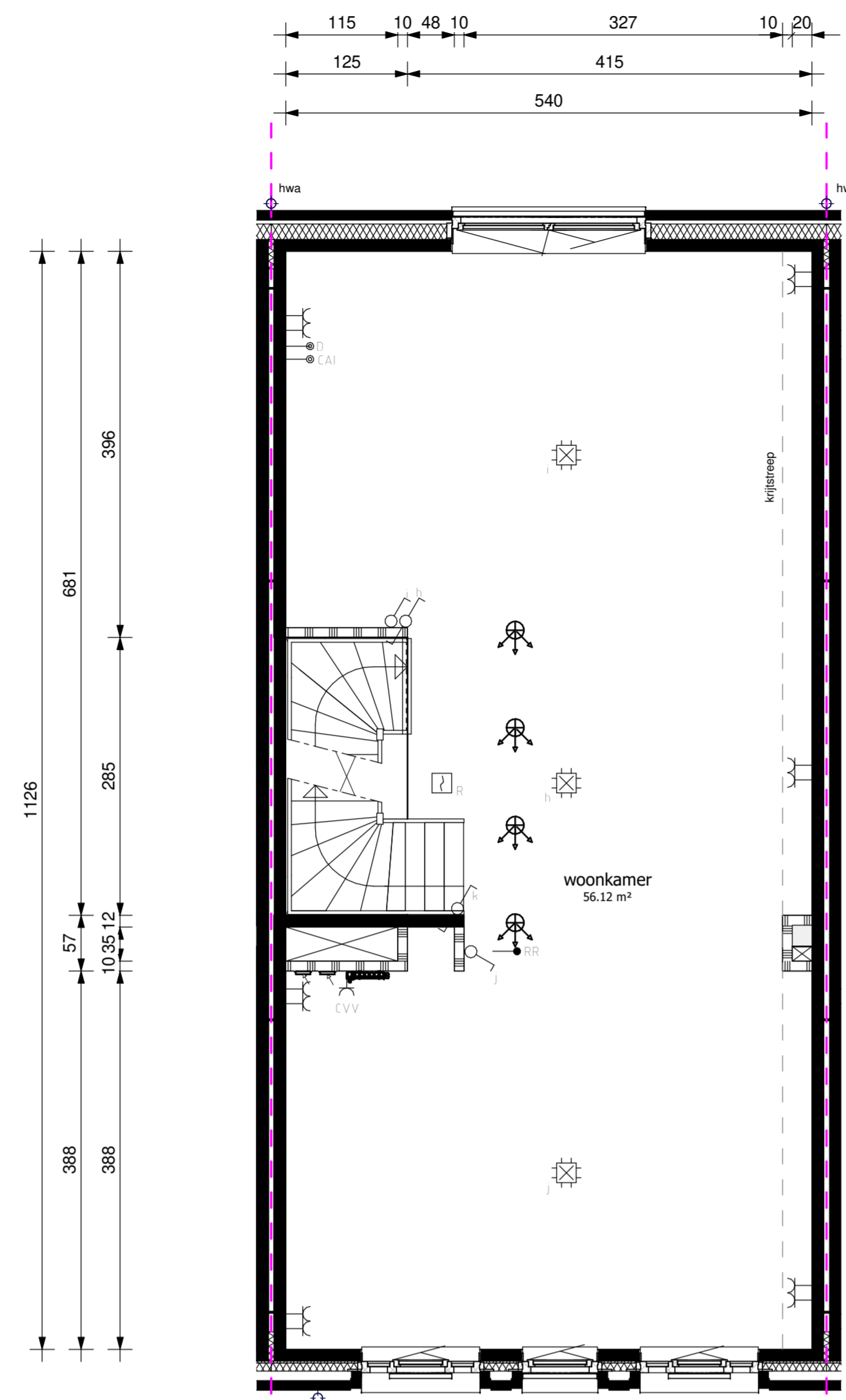
eerste verdieping
