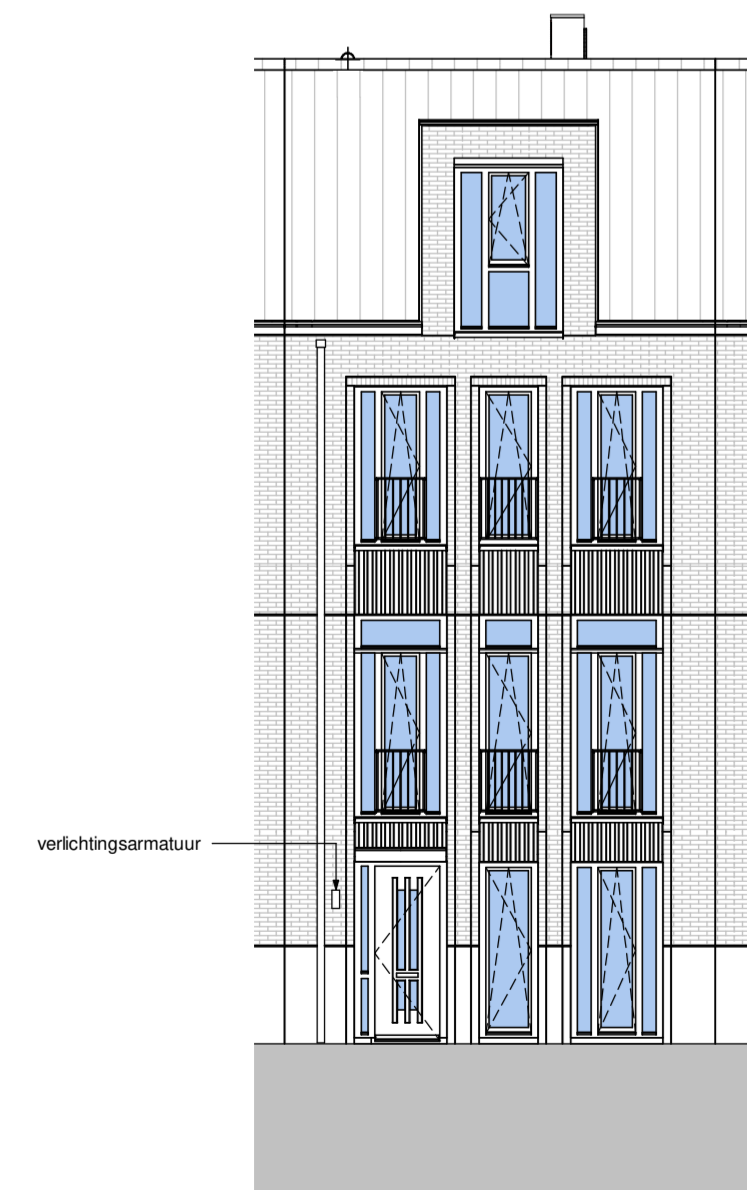
voorgevel
