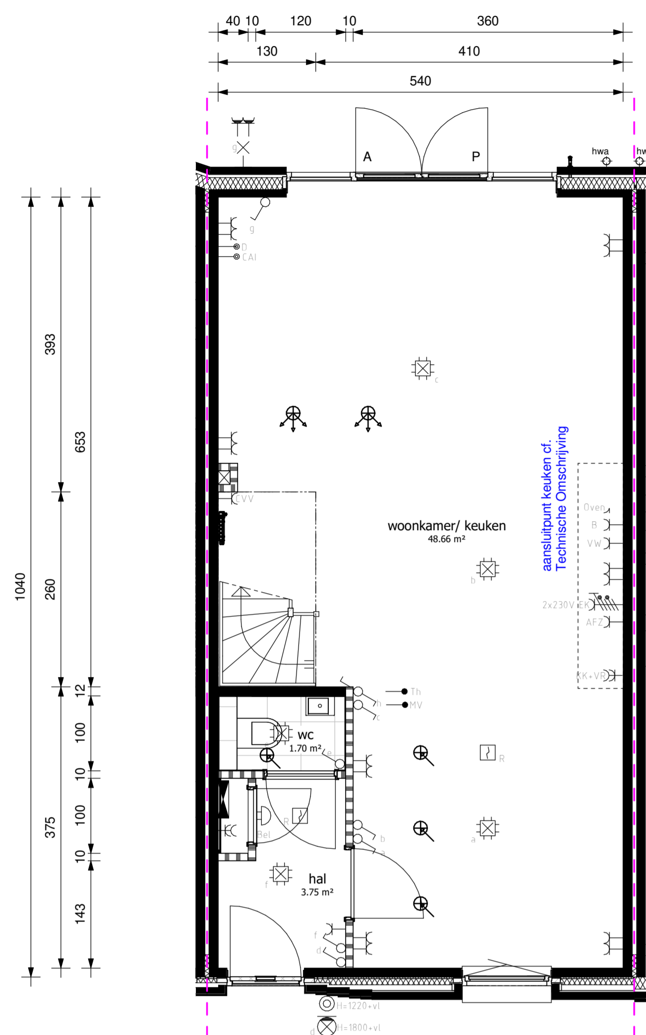
begane grond
